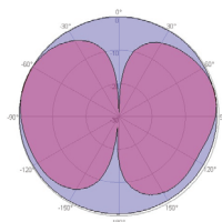
1710~2700MHz
