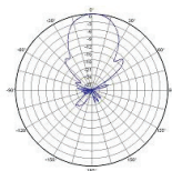
1710~2170MHz
