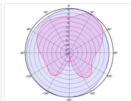
1710~2700MHz
