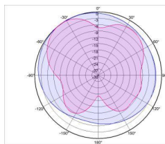
698~960MHz
