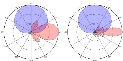
698~960MHz
