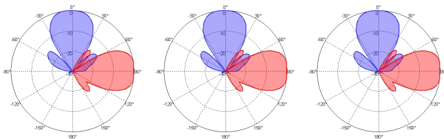
1710~2200MHz
